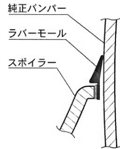
ラバーモール貼り付け要領(断面図)
